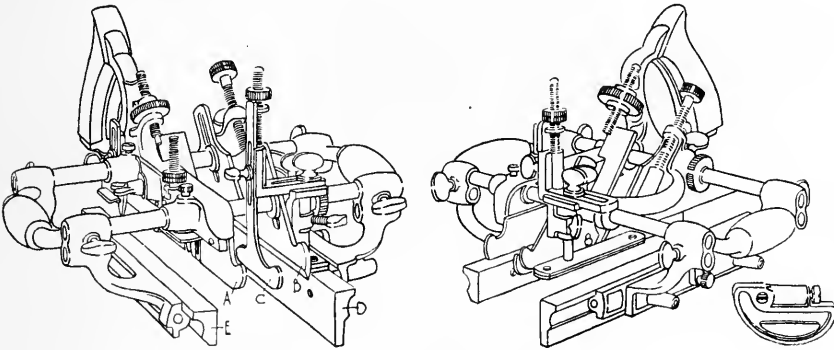
FIG. 73. UNIVERSAL PLANE.
